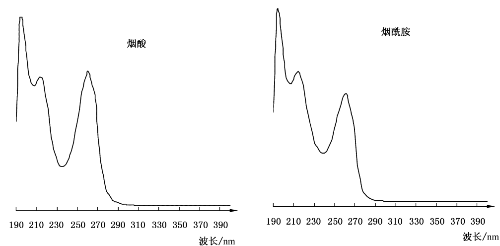
图 A.3 标准物质紫外吸收光谱图
