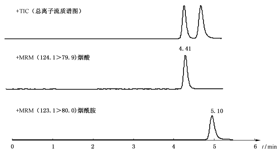
图 A.4 标准物质总离子流质谱图和提取离子(定量)质谱图
